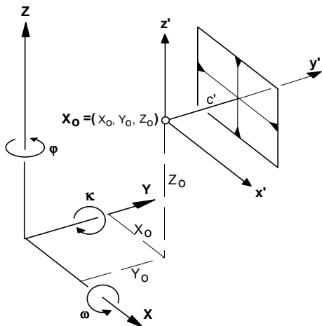
Abb. 3: Terrestrische Drehwinkel
